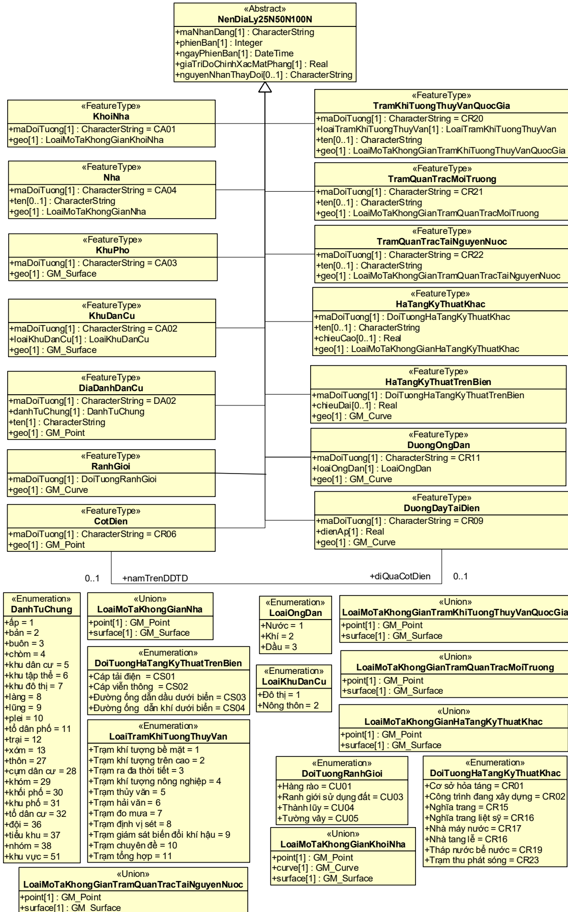
Hình 7. Lược đồ ứng dụng mô tả các lớp đối tượng địa lý trong gói dữ liệu dân cư
