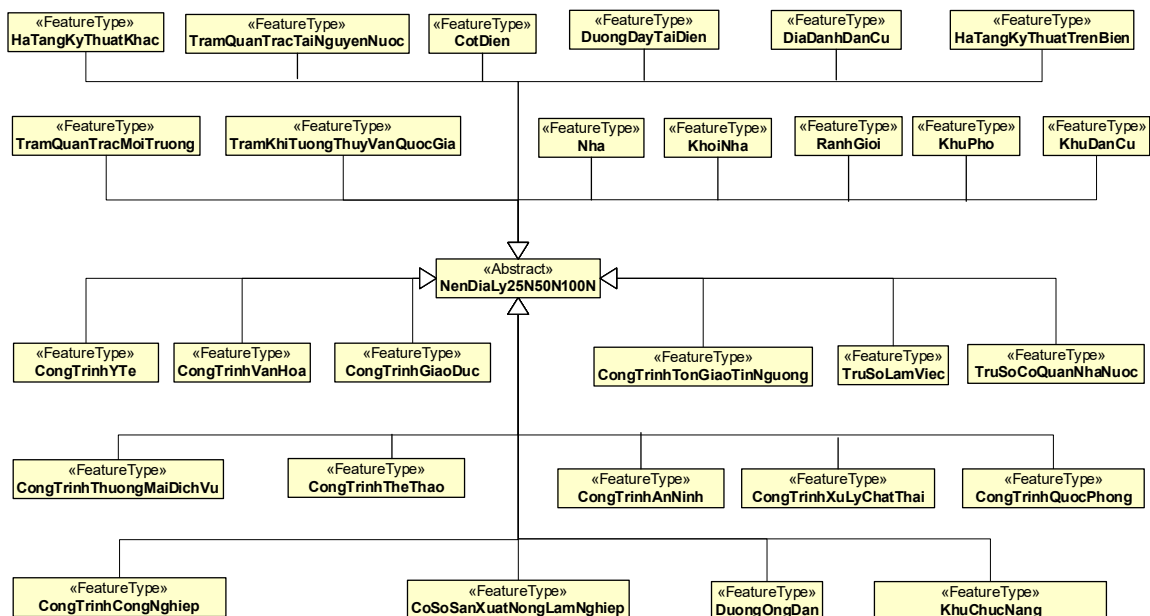
Hình 6. Mô hình đối tượng địa lý tổng quát gói dữ liệu dân cư
